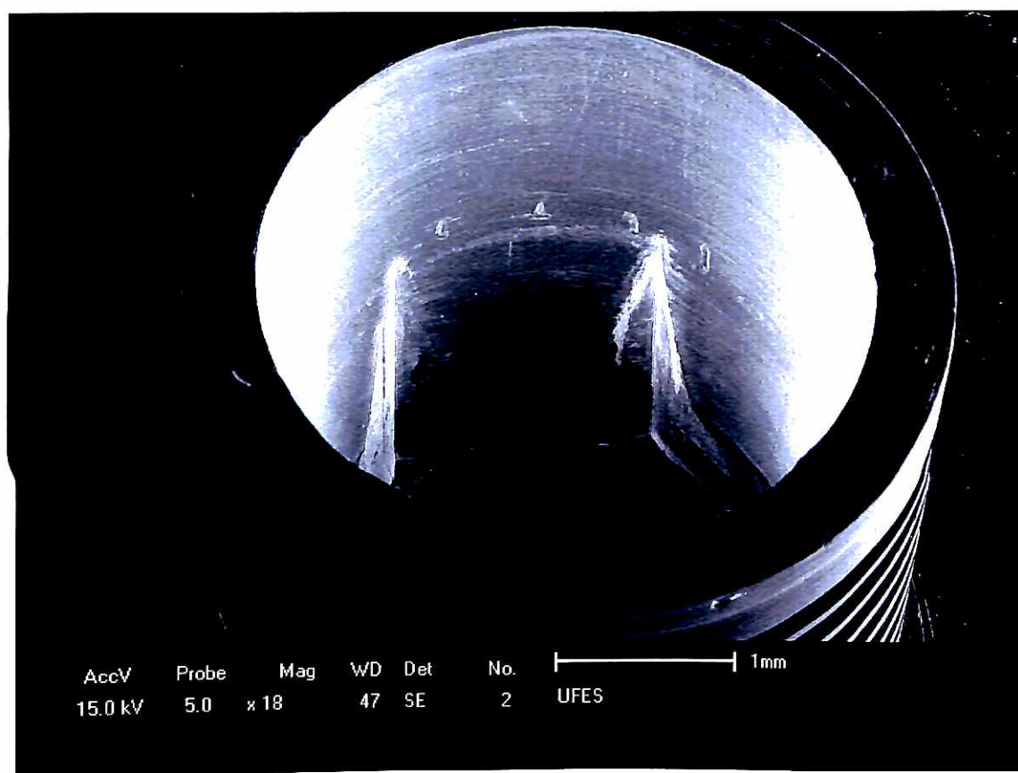
Figura 37 – Microscopia eletrônica de varredura: vista em 30° do oco do conjunto da Conexão®.
