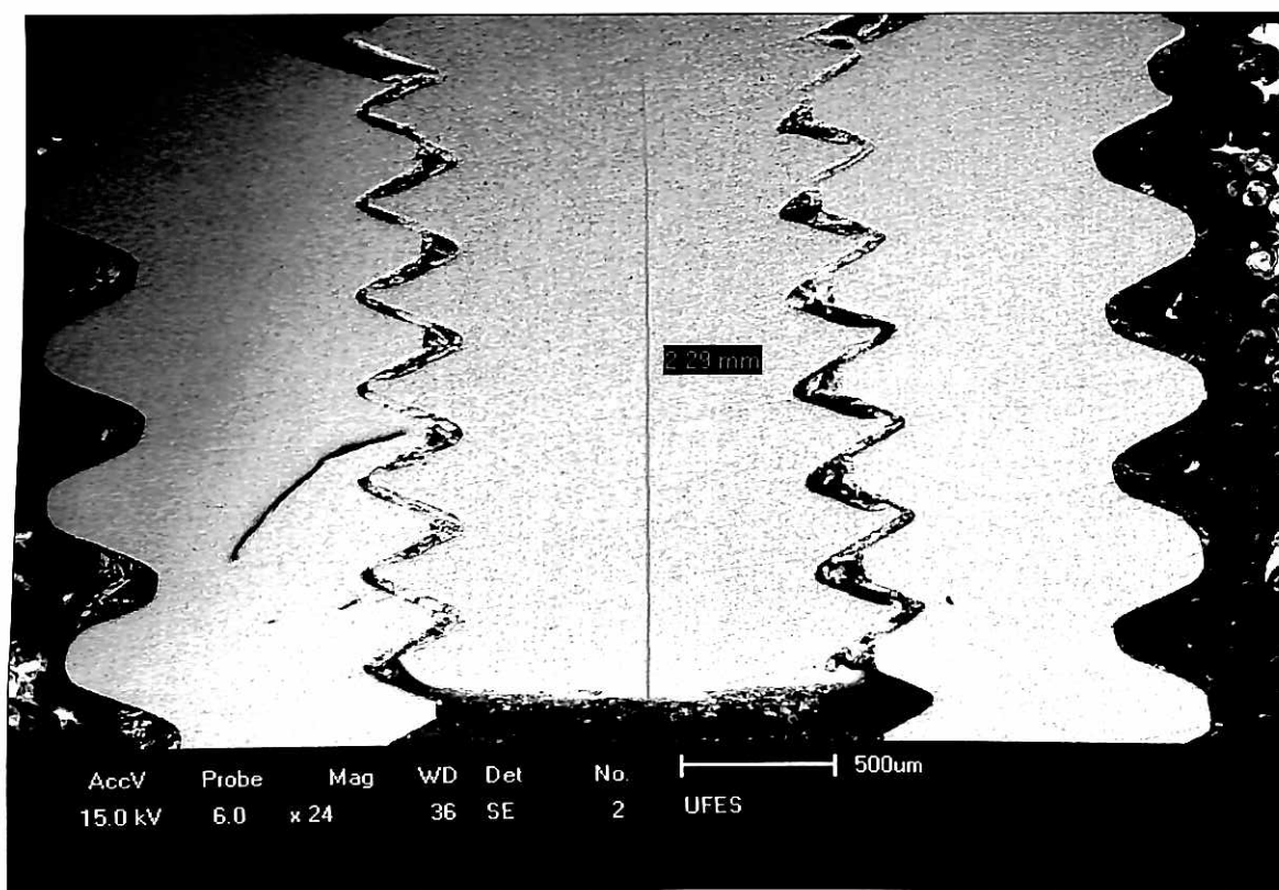
Figura 29 – Microscopia eletrônica de varredura: vista e medida da extensão do parafuso da Conexão® que penetra no oco do implante.
