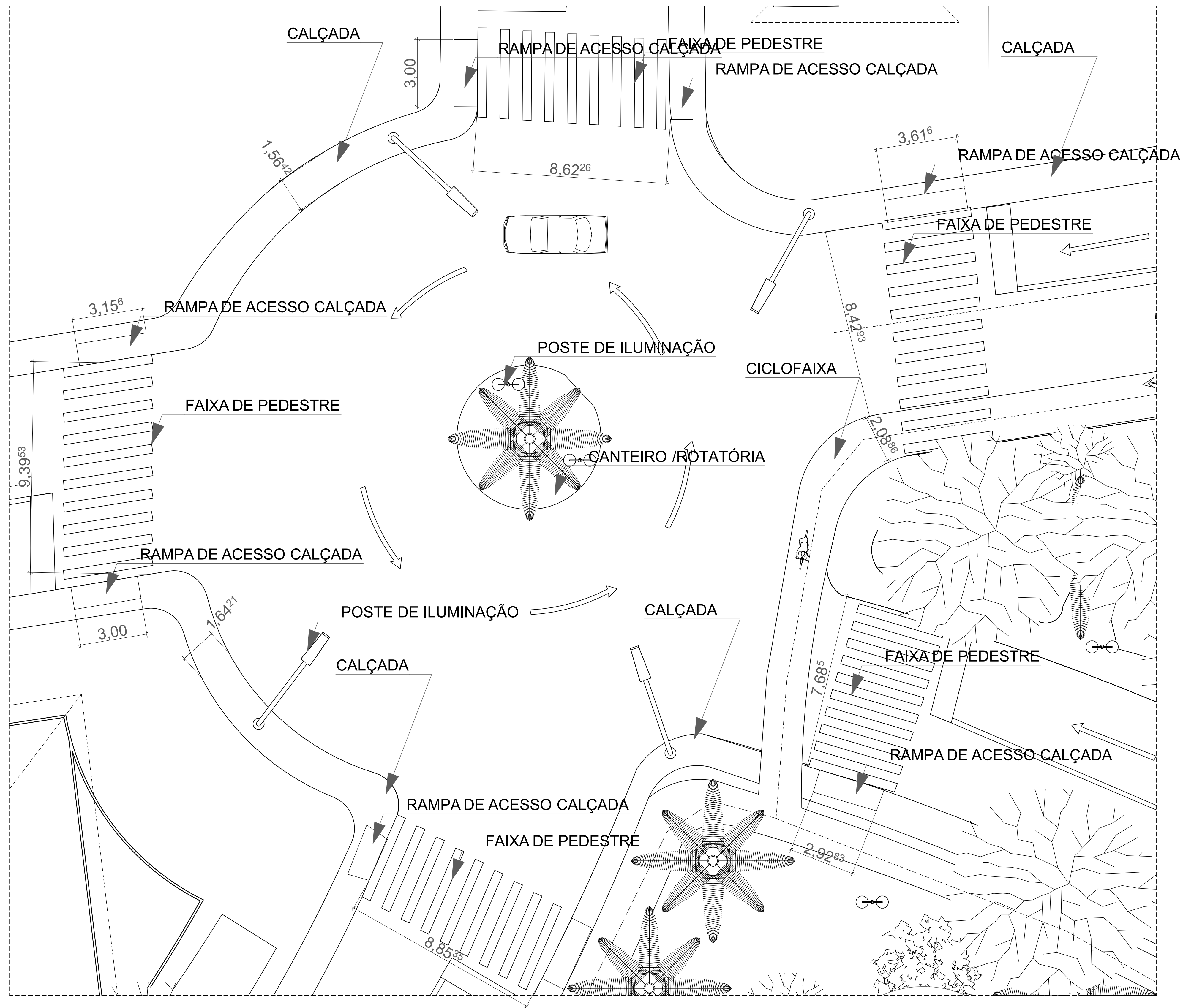
D-01 Det. Escala: 1:100
