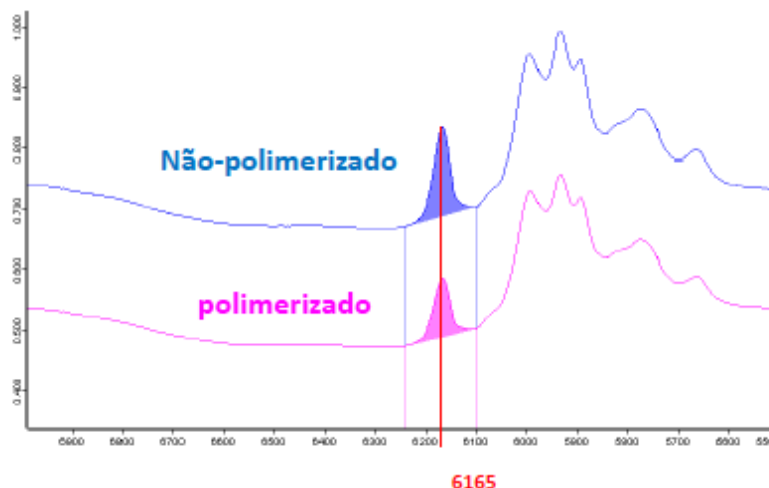
Figura 5: Espectro obtido no FTIR. Em azul a curva do material não polimerizado, e em rosa do material polimerizado. A área correspondente ao pico 6165\text{ cm}^{-1} correspondente à ligação vinílica foi calculada antes e após a polimerização.
