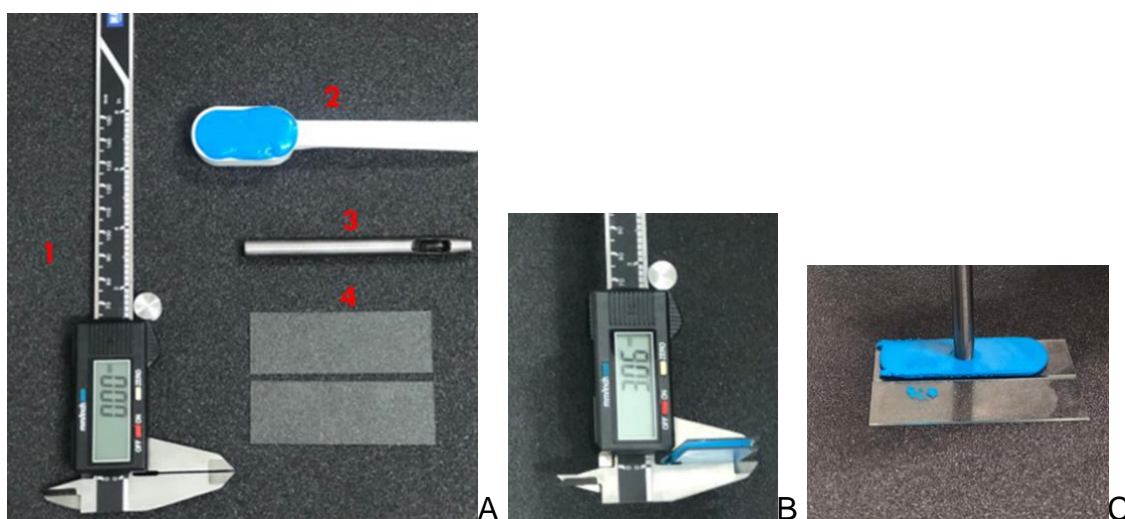
Figura 1: (A) Materiais para calibragem e confecção da matriz em silicone. 1. Paquímetro Digital, 2. Silicona de Condensação, 3. Punch com secção circular de 5mm, 4. Lâminas de vidro; (B) Calibragem da matriz de silicone; (C) Confecção do orifício com um Punch de 5mm de diâmetro interno.
