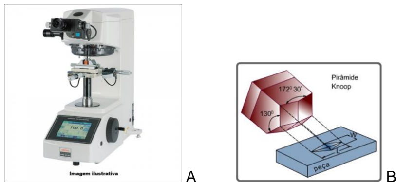
Figura 8: (A) Durômetro; (B) Indentador Knoop.
