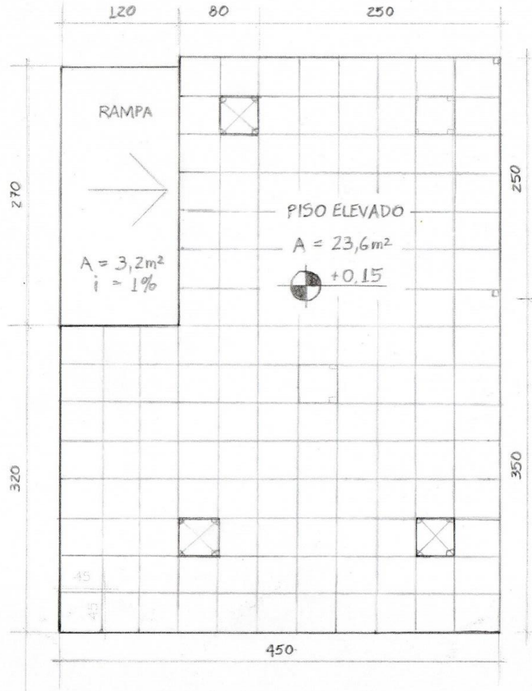
PLANTA PISO ESCALA 1:50
