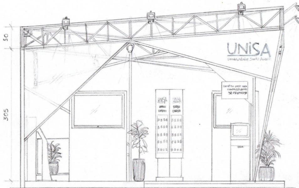
VISTA FRONTAL ESCALA 1:50
