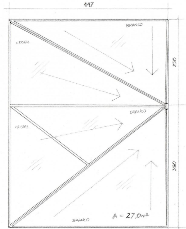
PLANTA COBERTURA ESCALA 1:50
