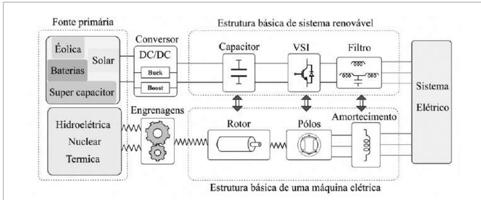
Figura 2.8 Estruturas básicas de um sistema renovável e de uma máquina síncrona.
