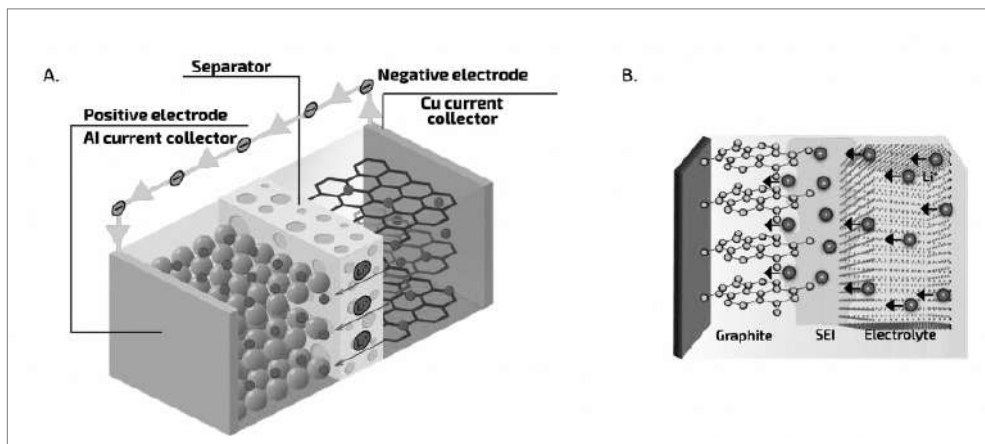
Figura 5.8 A) Bateria de Íon-Lítio durante a descarga. B) Formação da camada de passivação (SEI) no eletrodo negativo. Fonte: U.S. DOE, 2020.
