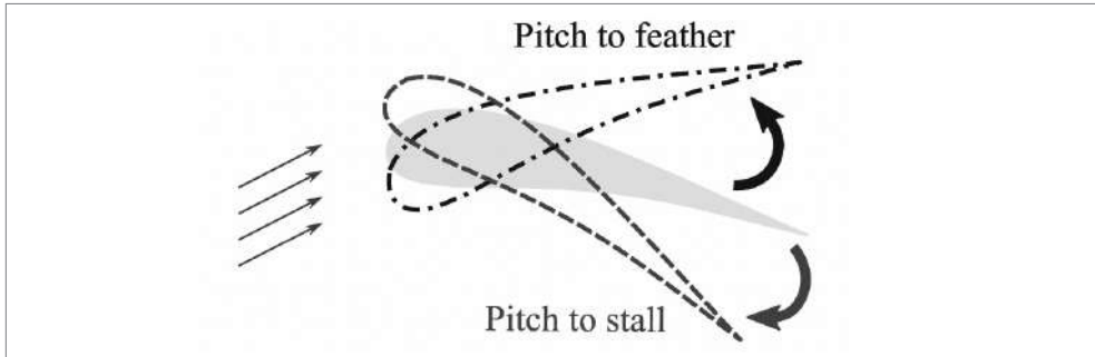
Figura 2.3 Controle de passo para o estol e para o embaeiramento.
