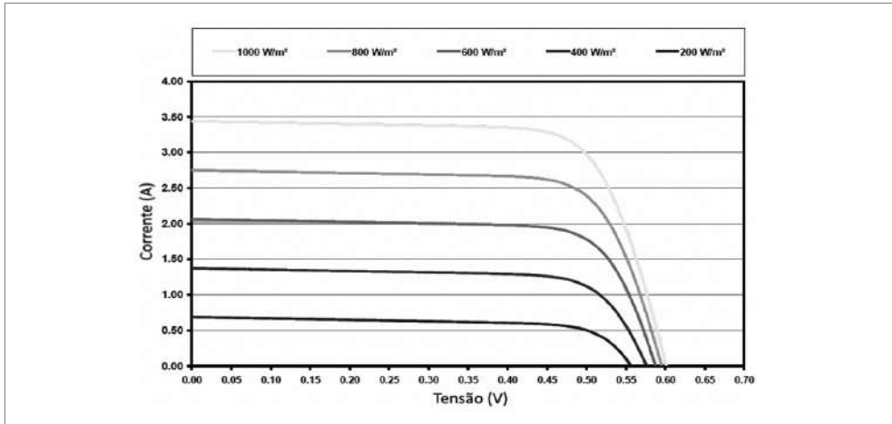
Figura 6.1 Curva corrente por tensão de uma fotocélula com diferentes irradiâncias.
