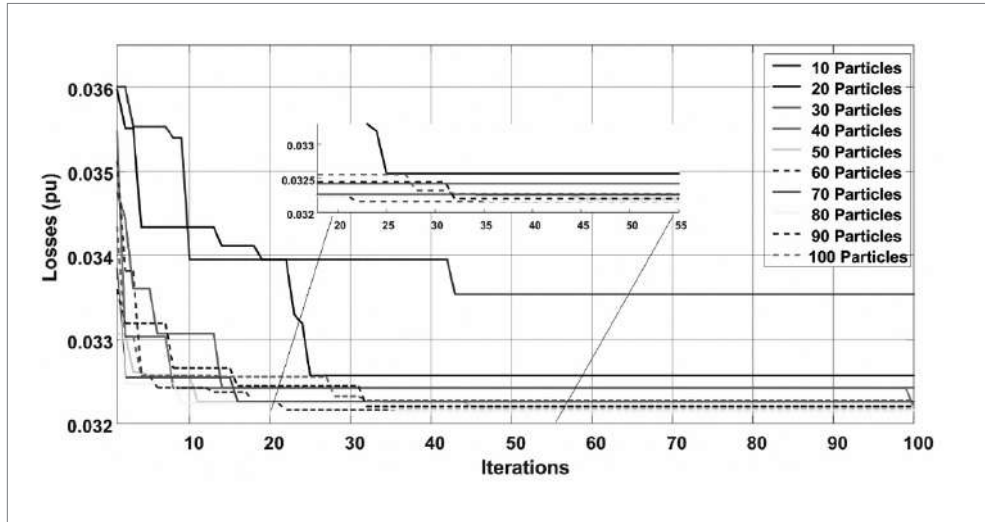
Figura 7.11 Convergência BPSO.
